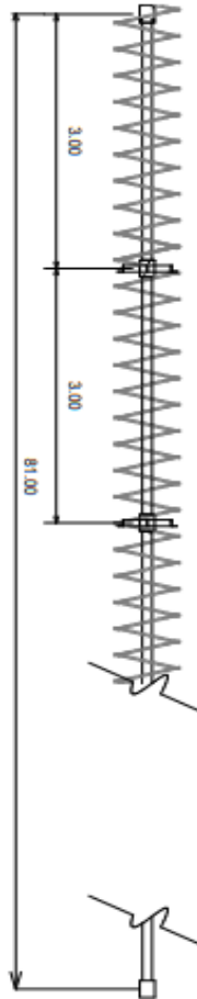
1 WALL PLAN 1 : 50
