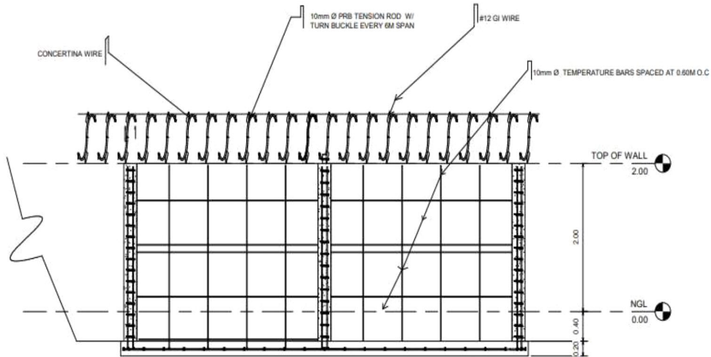
1 WALL DETAIL 1 : 30
